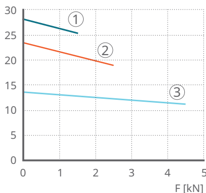
24 Geschwindigkeit-Last-Diagramm CAHB-20E
