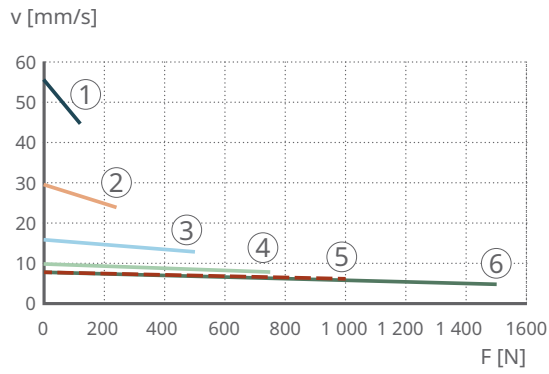
4 Geschwindigkeit-Last-Diagramm CAHB-10
