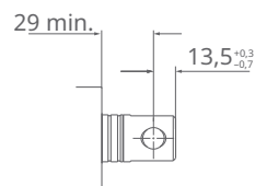
☐ 67 Vordere Befestigung mit Verdrehsicherungsrohr
