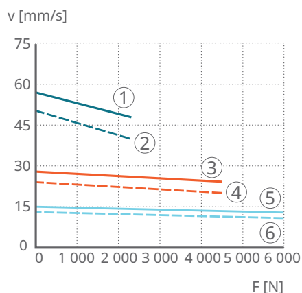
103 Geschwindigkeit-Last-Diagramm CAHB-31N
