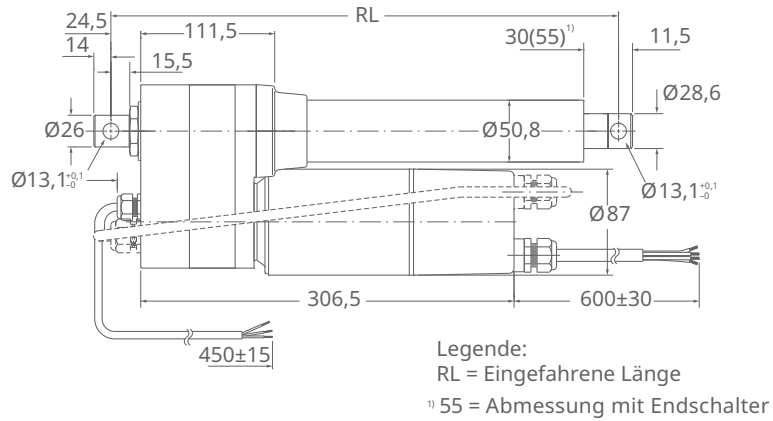
89 Seitenansicht optionales Potentiometer (gestrichelte Linie für optionalen Endschalter)
