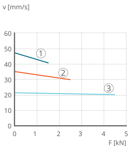
34 Geschwindigkeit-Last-Diagramm CAHB-21S
