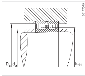
Anschlussmaße
