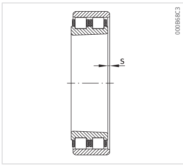
Axialer Verschiebeweg
